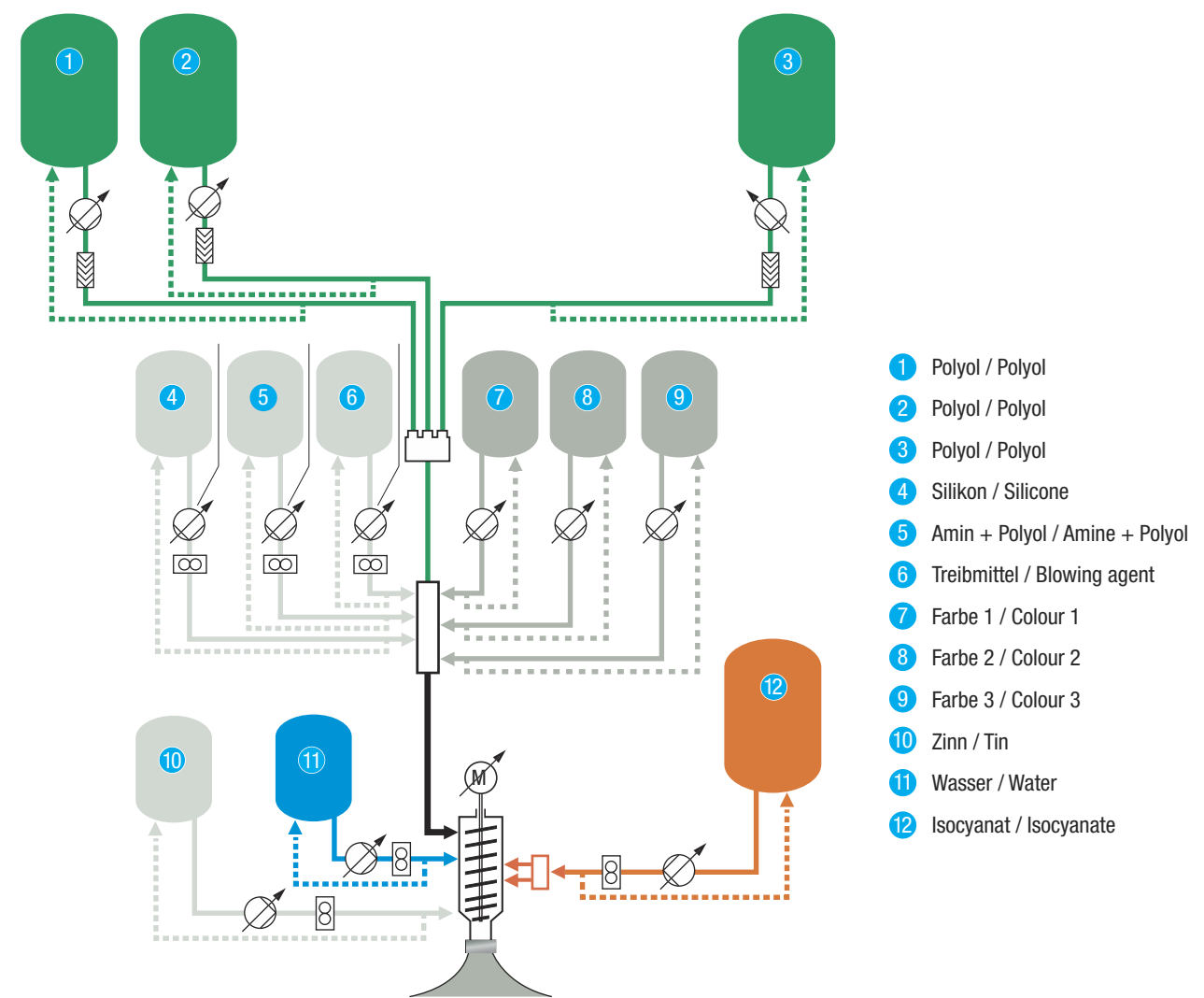
Schema einer QFM-Standard-Dosiereinheit Schematic diagram of a QFM standard metering unit
